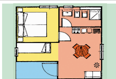
Bungalow bilocale Tipo A - mq. 22 + veranda con gazebo. Prefabbricato in cemento precompresso, soggiorno con angolo cottura + frigo basso, nel soggiorno una rientranza senza porta con letto singolo, camera con letto matrimoniale, bagno con doccia e climatizzazione. Senza TV e cassetta di sicurezza.
